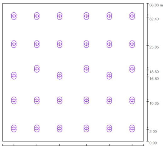
(照明数量及び配置) 5000K30台, 3000K30台
