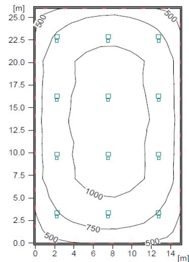
(LED 予想照度) 480W 12台, 150W 12台 眩しさ防止つき
