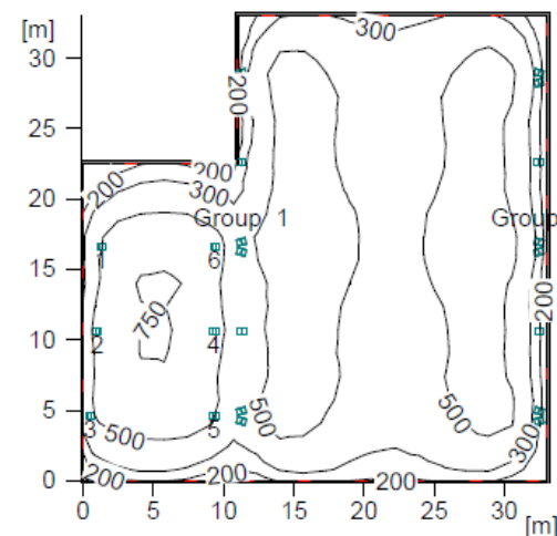
(LED 予想照度) 320W 22台 眩しさ防止つき
