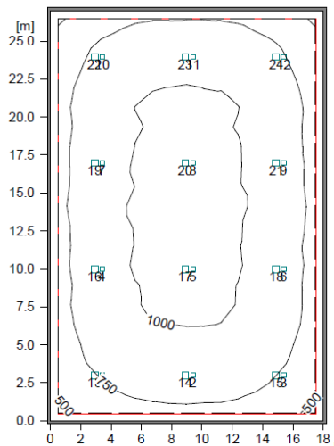
既存照明 メタハラ1000W 12台, ナトリウム180W 12台
