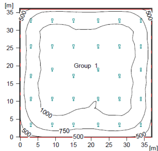
(LED 予想照度) 480W 30台, 150W 30台 眩しさ防止つき
