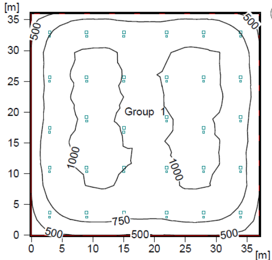
既存照明 メタハラ1000W 30台, ナトリウム180W 30台
